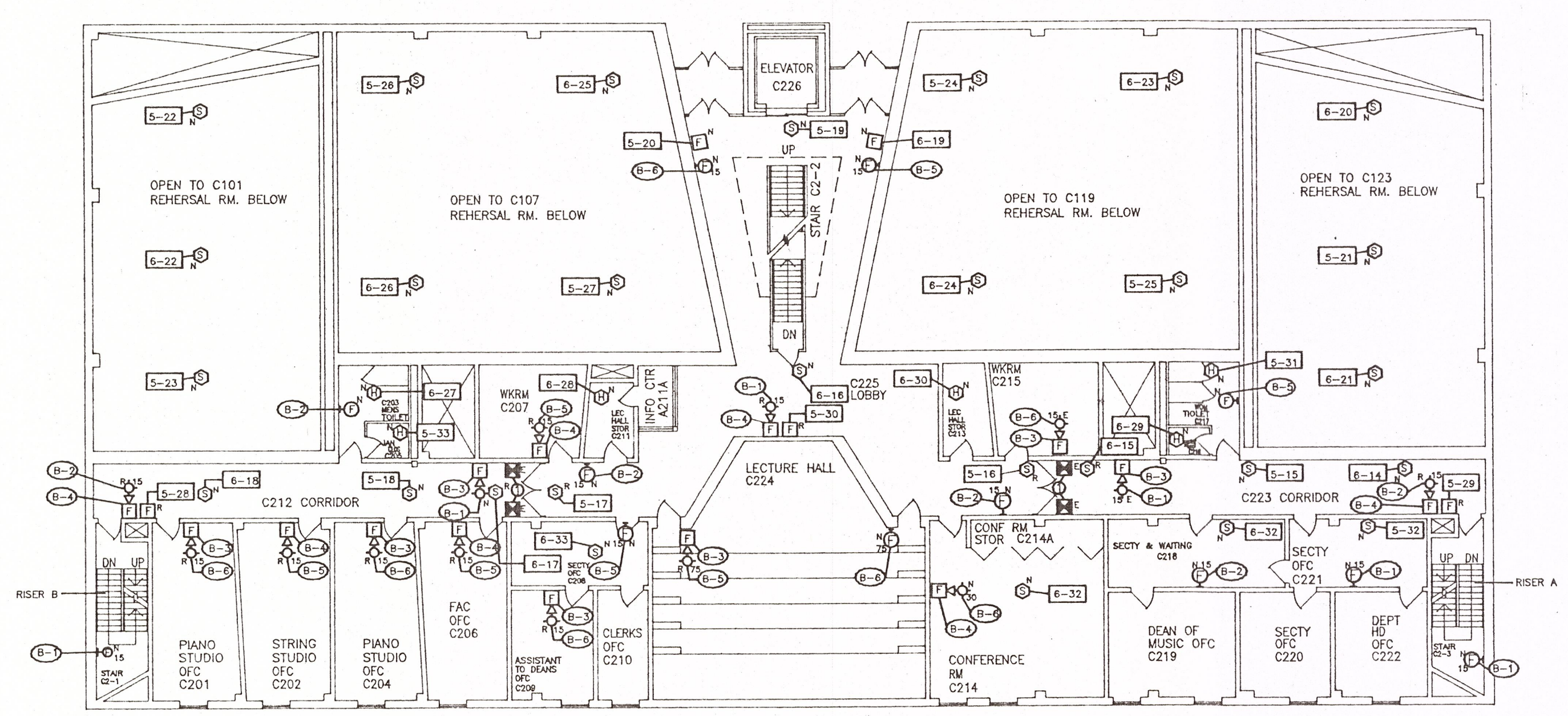
2 PLAZA PLAN - LEVEL 2 A5 SCALE: 1/16" = 1'-0"
