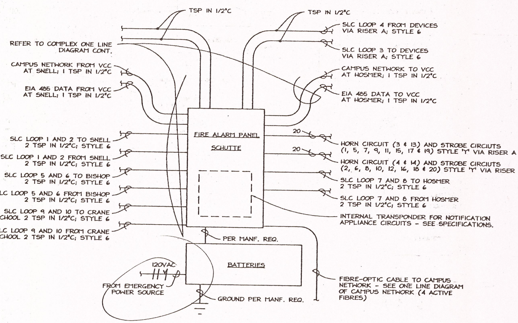
DETAIL - FIRE ALARM PANEL N.T.S.
