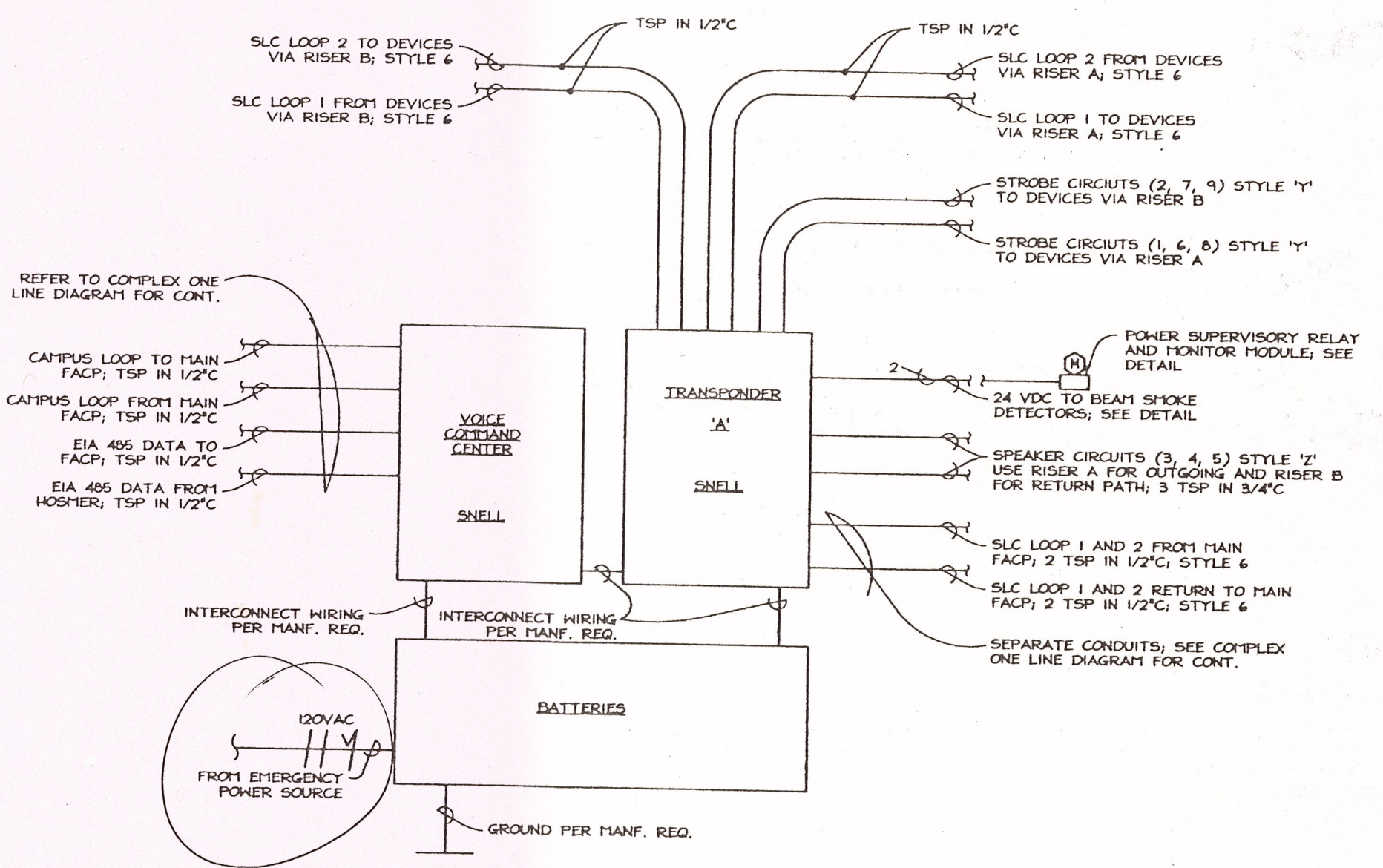
DETAIL - TRANSPONDER 'A' N.T.S.
