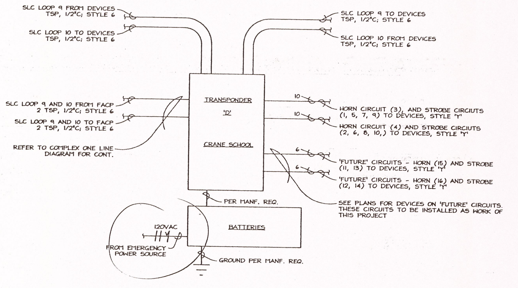
DETAIL - TRANSPONDER 'D' N.T.S.
