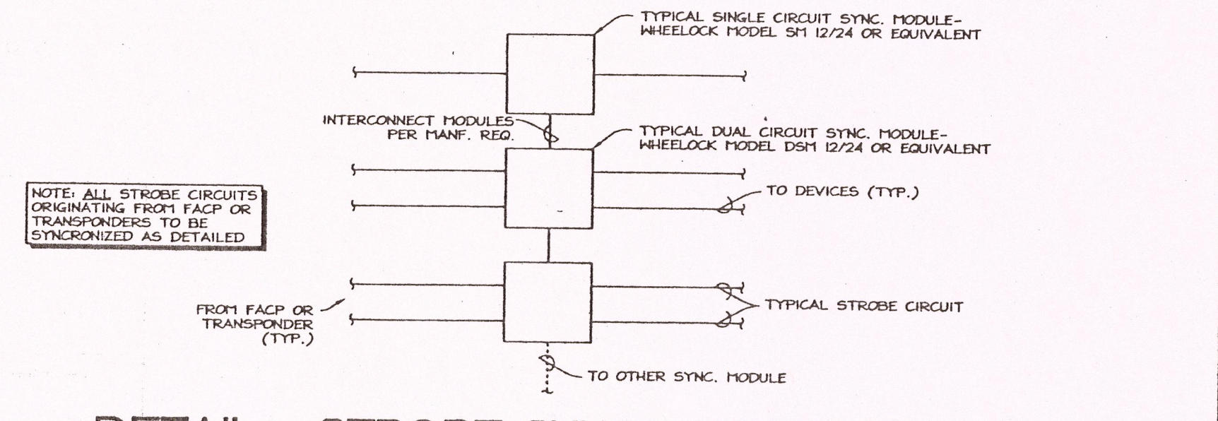
DETAIL - STROBE SYNCHRONIZATION N.T.S.
