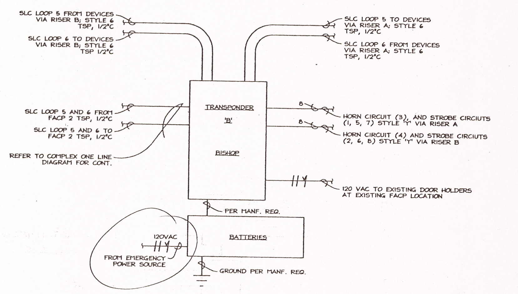
DETAIL - TRANSPONDER 'B' N.T.S.
